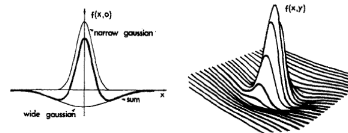
(Rodieck 1965)
