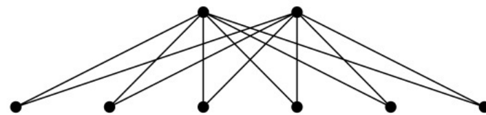
K_{2,6}
